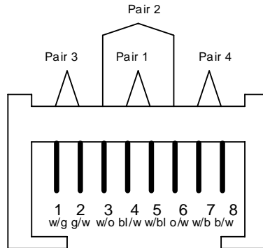
T 568-A
